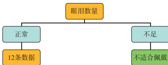
图 2.3.5 隐形眼镜决策树的第一层
