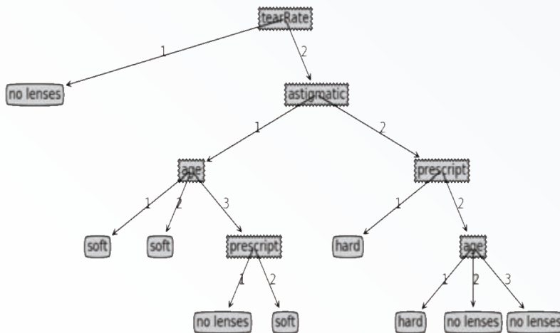
图 2.3.7 借助 Python 编程语言绘制的决策树
