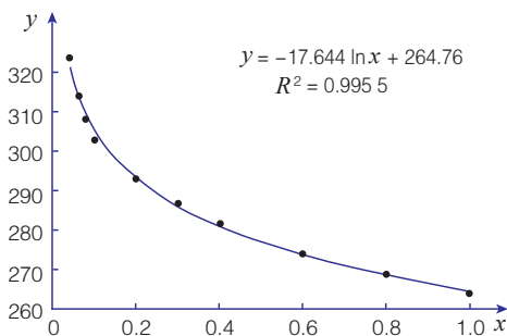
图2.2.5 非线性回归问题趋势线图
