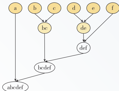
图 2.4.7 基于层次的聚类
