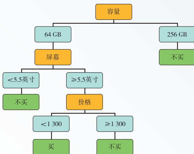
图 2.3.2 手机选择决策树
