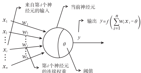
图 2.5.3 M-P 神经元模型
