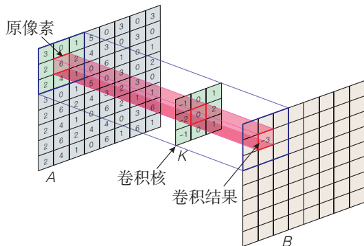
图 2.5.14 二维卷积过程
