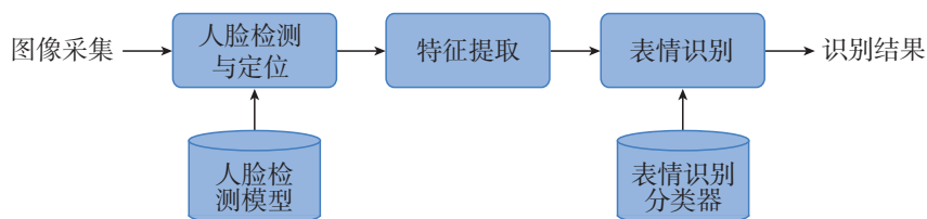
图 3.1.3 表情识别的基本流程示意图
