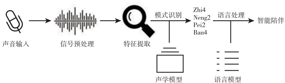
图 3.2.9 语音识别技术流程示意图
