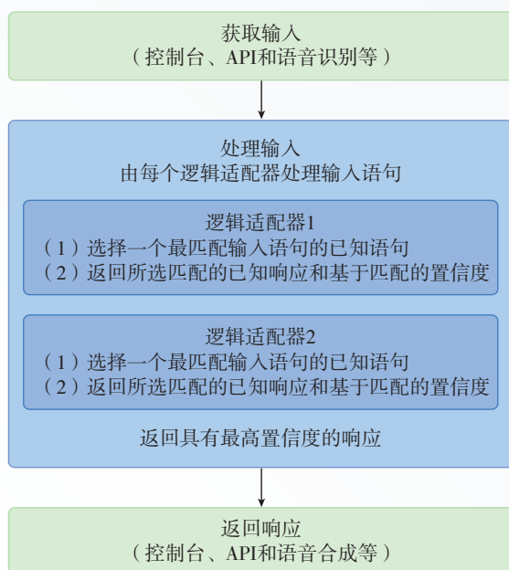
图3.2.7 ChatterBot的处理流程图
