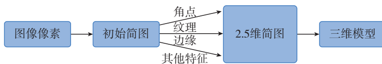
图3.1.2 马尔视觉计算过程示意图
