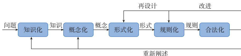
图 2.1.10 构建专家系统的一般流程示意图
